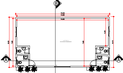
PLANTA BAIXA ESC.: 1/200
